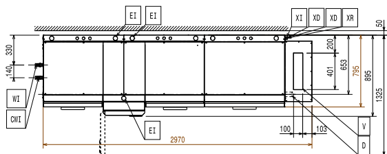
Dessus
