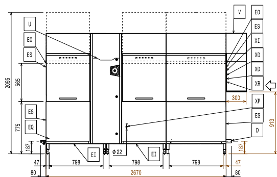
Côté
